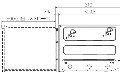
側面図
