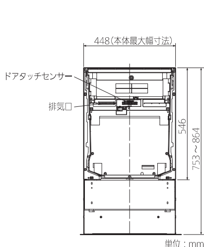
正面図
