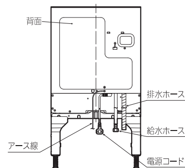
背面図
