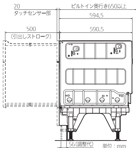
側面図
