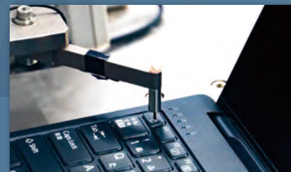
キーボードたわみ試験
