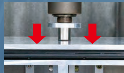
天板からの全面加圧試験(約200kgf)
