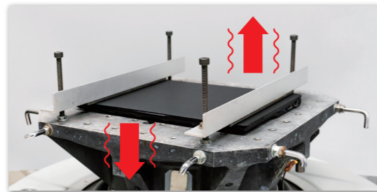
振動試験&衝撃試験
