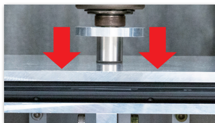
天板からの 全面加圧試験 (約200kgf)
